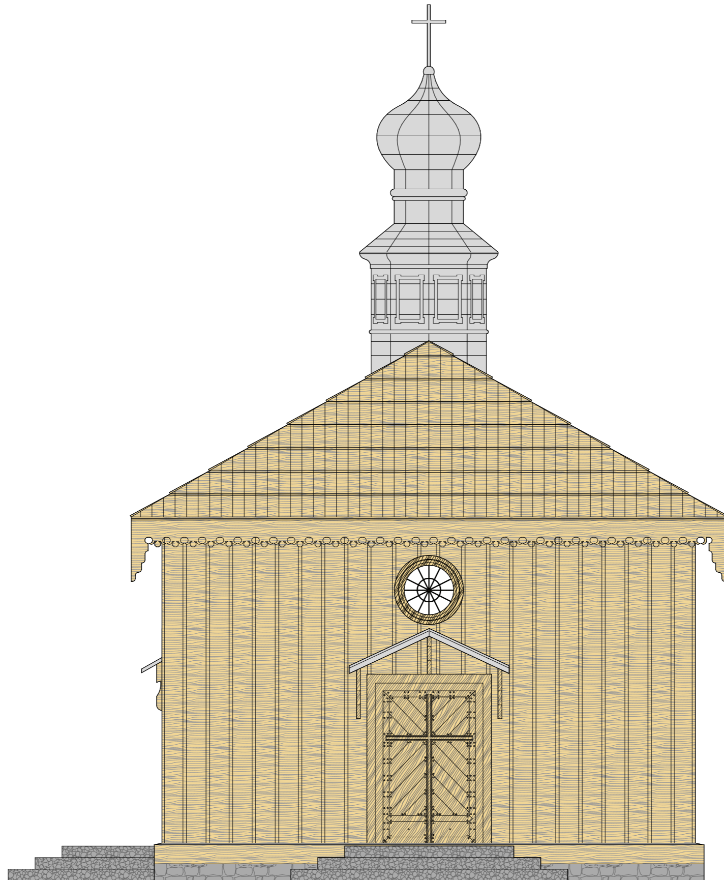
ELEWACJA ZACHODNIA SKALA 1:50
