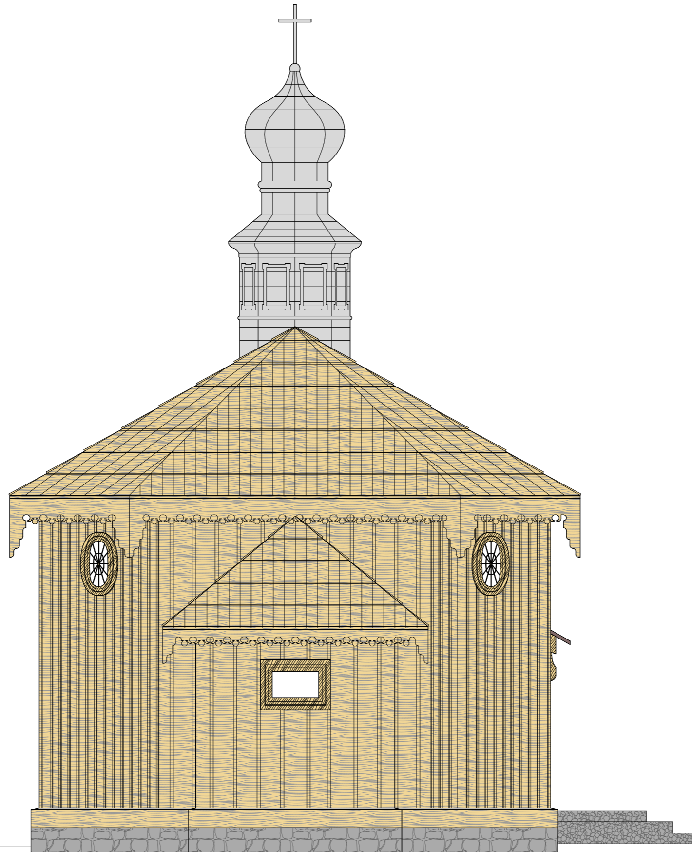
ELEWACJA WSCHODNIA SKALA 1:50
