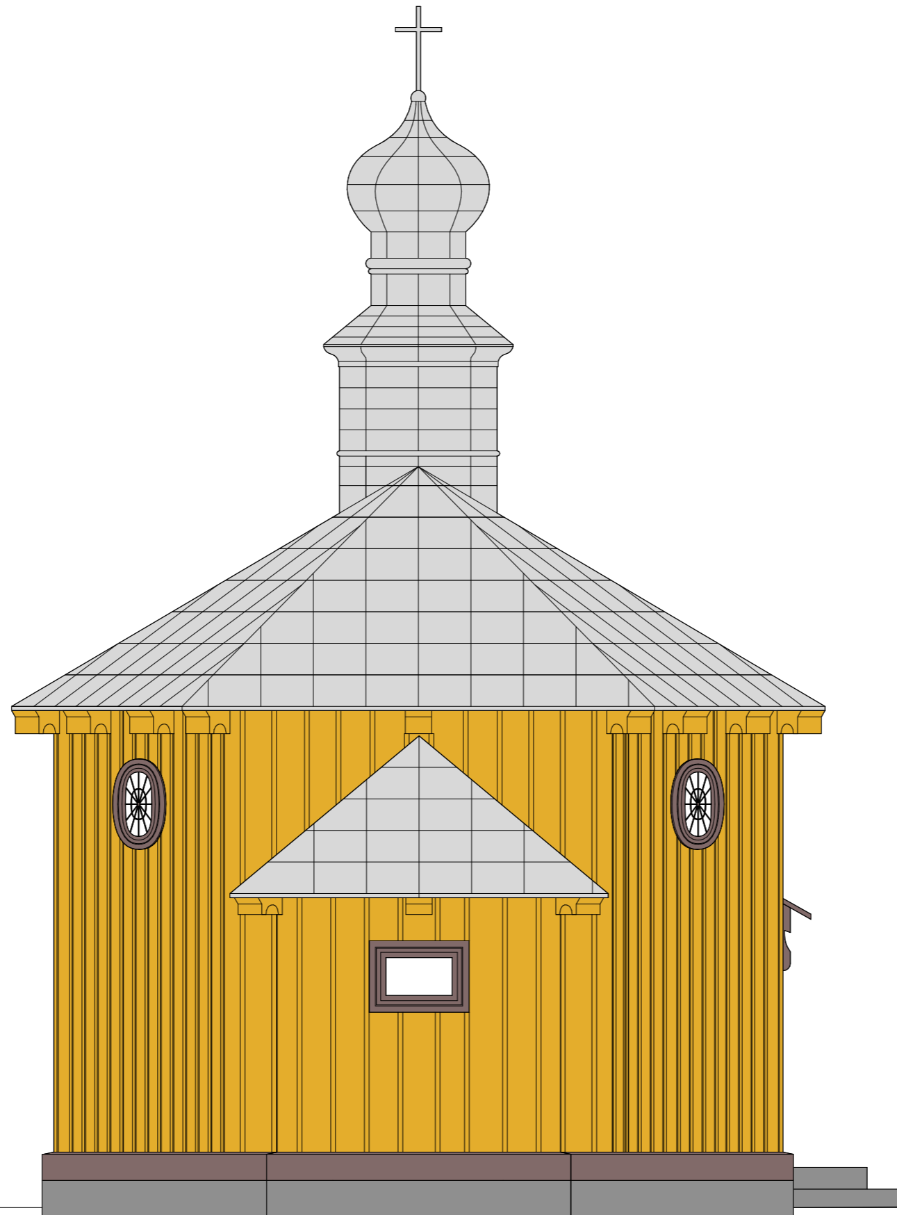
ELEWACJA WSCHODNIA - INWENTARYZACJA SKALA 1:50
