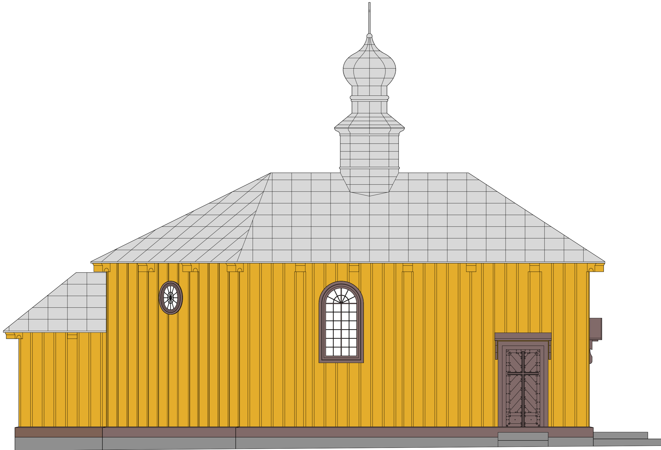
ELEWACJA PÓLNOCA - INWENTARYZACJA SKALA 1:50
